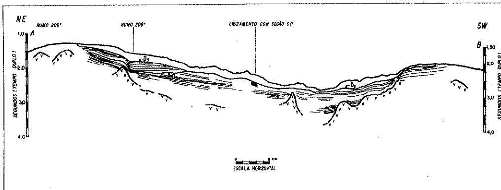
Figura 2 — Seção sísmica AB , através do Platô de Pernambuco, paralela à costa. D_1 e D_2 são interpretadas como superfícies de erosão
