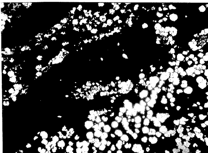
Foto 3 — Fotomicrografia de lâmina delgada. Minério oxidado, onde os cristais de espessartita inalterados permanecem como relictos do protominério substituído. Nicóis paralelos. (Aumento 22 vezes)
