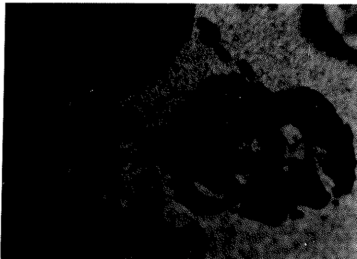
Foto 8 – Fotomicrografia de seção polida. Minério de substituição, com cristais semidissolvidos de espessartita, associados à litioforita. Nota-se a transformação da litioforita para nsutita cristalina. (Aumento 450 vezes)
