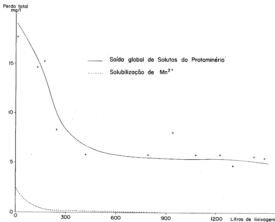
Figura 1 — Solubilidade dos piroxenóides (piroxmangita e rodonita) no decorrer do ensaio. A descontinuidade de solubilidade, verificada a 400 litros de lixiviação, corresponde à formação da crosta de alteração que recobre os minerais
