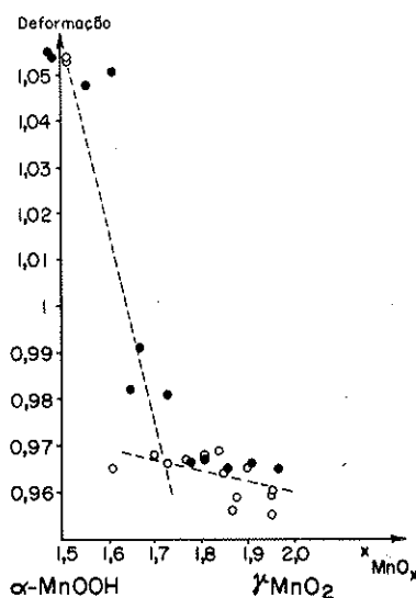
Figura 2 — Avaliação da deformação Jahn-Teller em função do estado de oxidação do manganês. Os círculos cheios foram obtidos na redução de MnO_2 (Bernhard) e os círculos vazios na oxidação de MnOOH (Leuenberger). O valor 1 corresponde a um octaedro regular
