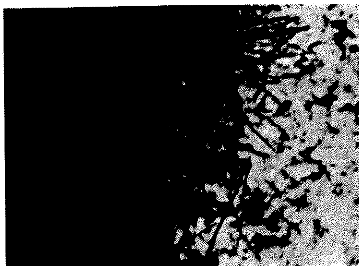
Foto 6 — Fotomicrografia de lâmina delgada. Agulhas bem cristalizadas de manganita no interior da crosta de alteração dos piroxenóides. Nicóis paralelos. (Aumento 100 vezes)
